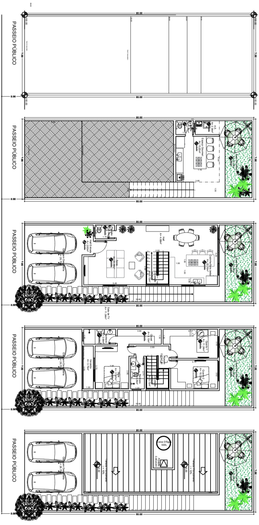
PLANTA PLANALTIMÉTRICO esc. 1:100
